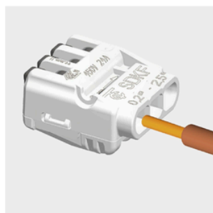
Für eindrängige Leiter ist es nicht notwendig den Hebel vor dem Einstecken des Leiters zu öffnen
