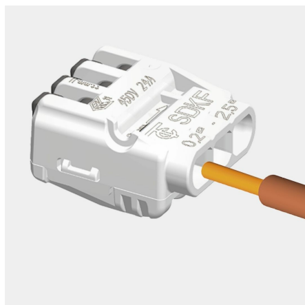
Für eindrähtige Leiter ist es nicht notwendig den Hebel vor dem Einstecken des Leiters zu öffnen
