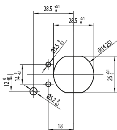
KADO 2/3 OS | Blechstärke | Plate thickness 0.5 – 1.0 mm | PH2 - 1,2 Nm
