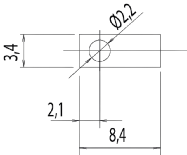
Cutout
