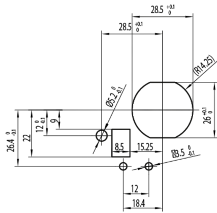
KADO 2/3 EE OS | Blechstärke 0,5 – 1,0 mm | PH2 - 1,2 Nm
