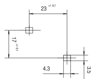
Lochbild
