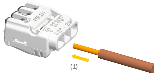
Für starre Leiter ist es nicht notwendig, den Hebel vor dem Einstecken des Leiters zu öffnen For rigid wires it is not necessary to open the lever before pushing in the wire
