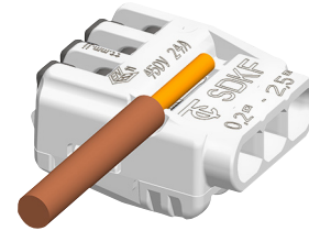
Messhilfe für Abisolierlänge Gauge wire skinning length
