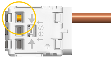
Kontrollfenster für korrekt abisiolierte und eingesteckte Leiter Control window for correctly skinned and pushed-in wires
