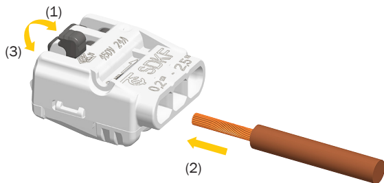
Bei flexiblen Leitern Lösehebel öffnen/schließen For flexible wires open/close the release lever
